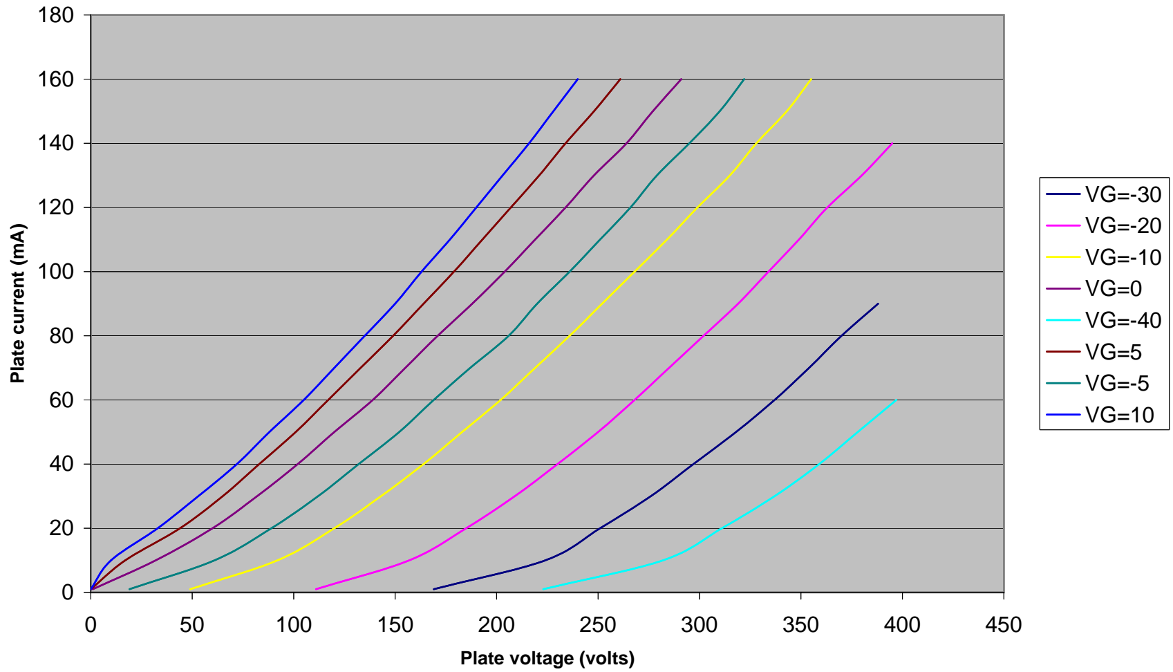
PT15 Triode mode (G2=G3=A)
