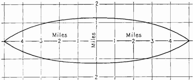
FIG. 100.—Fan pattern of the fan marker.
